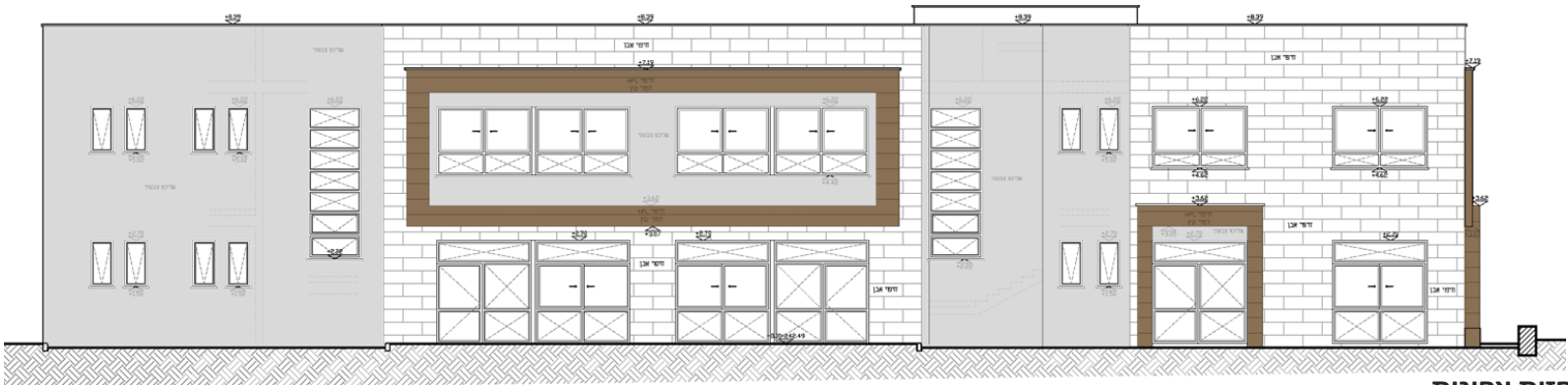
חזית צפונית
